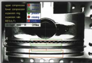
Vérification des tolérances
